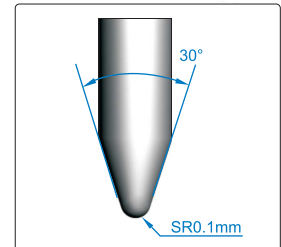
HS5D indenter
